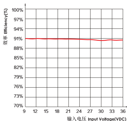
效率VS输入电压 (满载)
