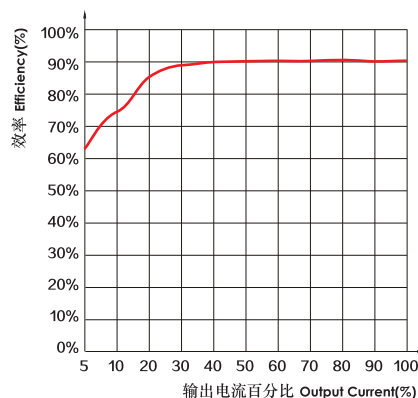
效率VS输出负载 (Vin=9-36VDC)
